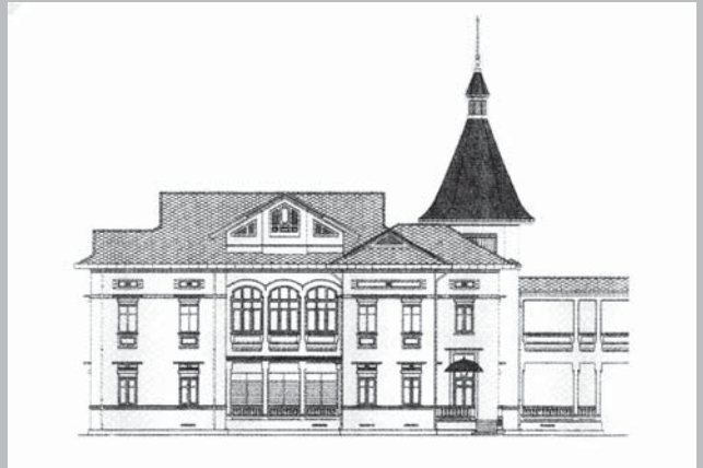
แบบพระที่นั่งศรีสุทธินิवास
